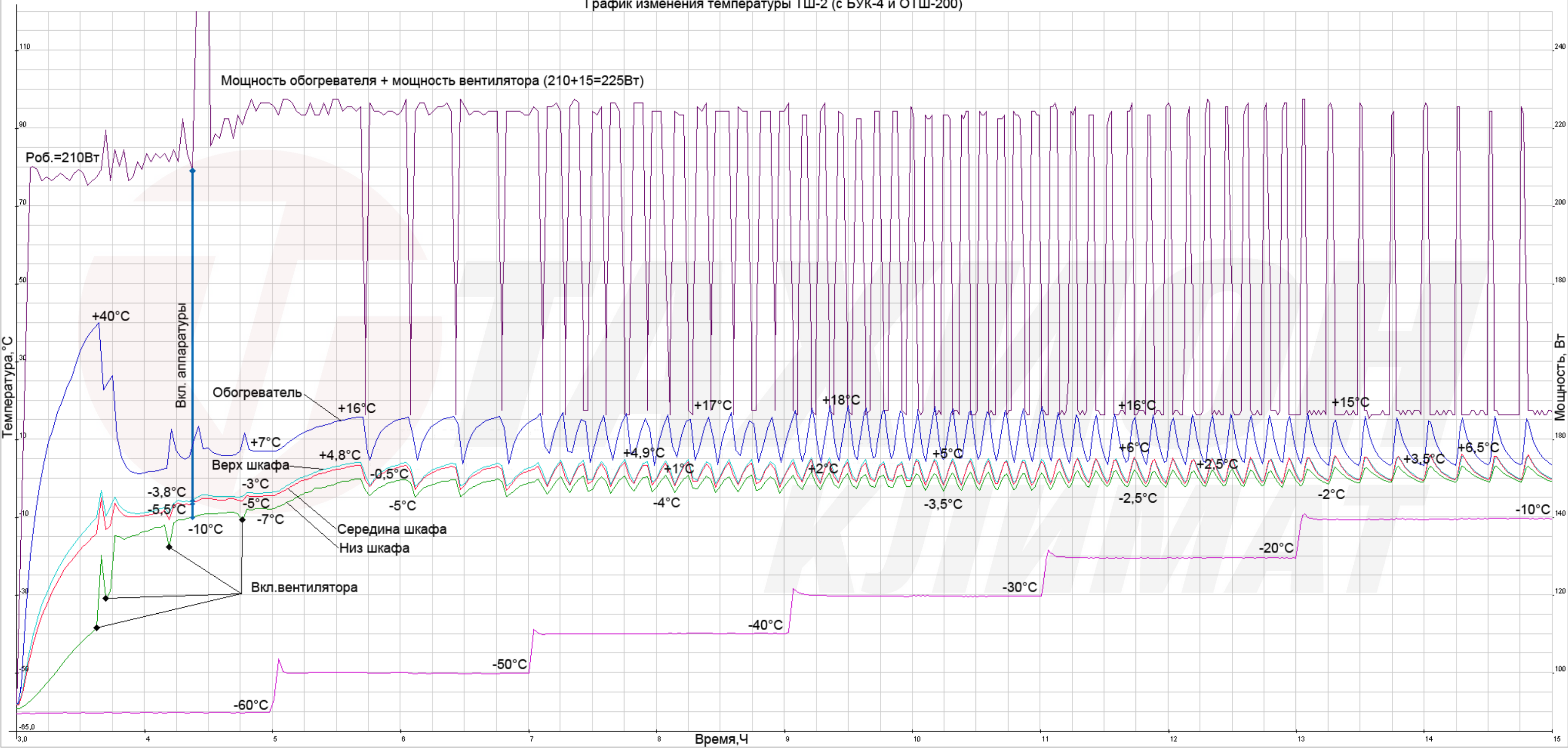
График изменения температуры ТШ-2 (с БУК-4 и ОТШ-200)
