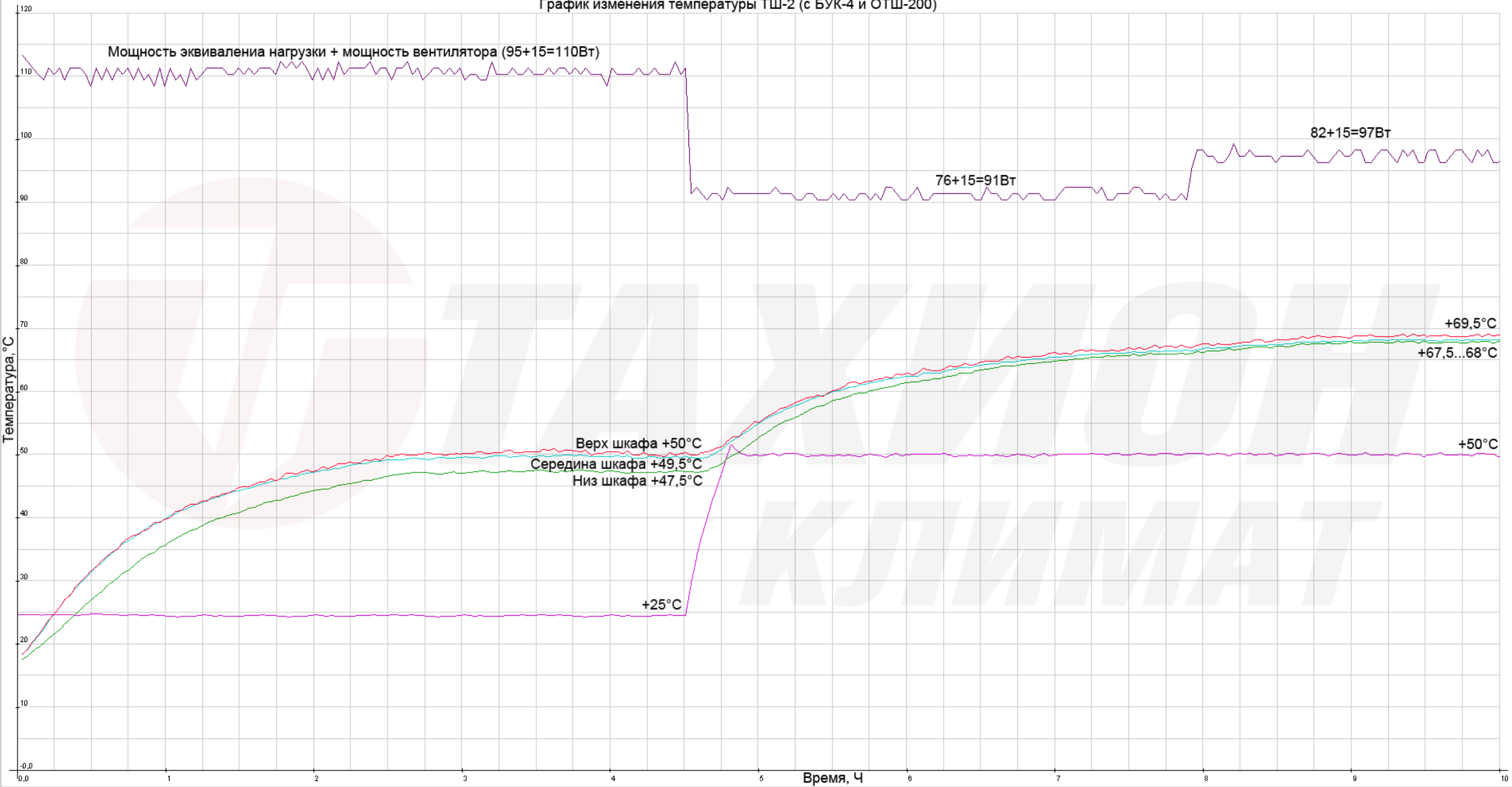
График изменения температуры ТШ-2 (с БУК-4 и ОТШ-200)
